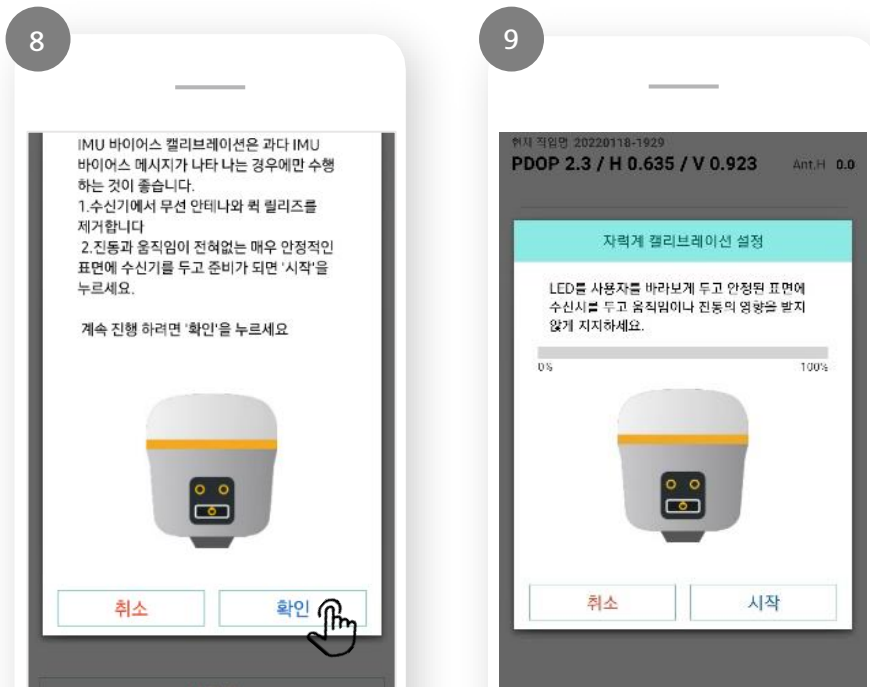
내용 확인 후 [확인] 클릭 -IMU 바이어스 보정은 과다 IMU 바이어스 메시지가 나타나는 경우에만 수행하는 것이 좋습니다.
