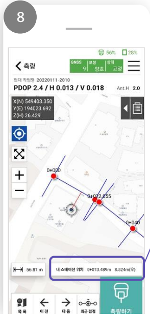
도로 중심선을 기준으로 내 스테이션 위치를 확인
