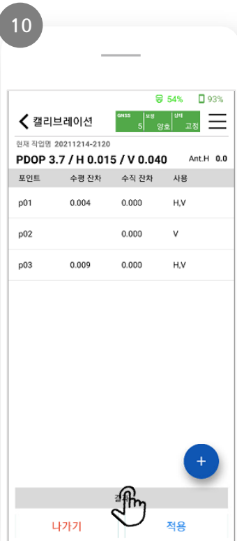
포인트 4점 추가 시 캘리브레이션의 결과 확인 가능 - 수평잔차/수직잔차의 값을 확인 후 양호한지 확인합니다.
