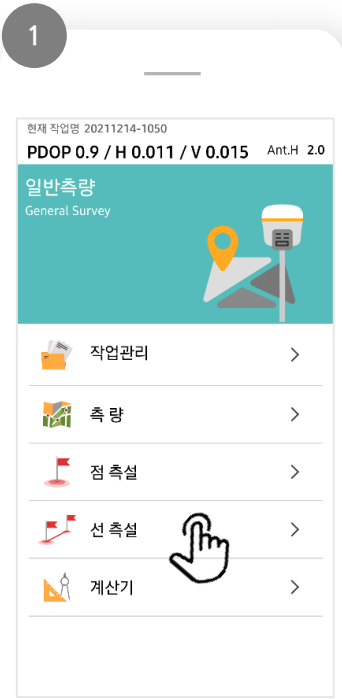
[일반측량-선 측설] 클릭
