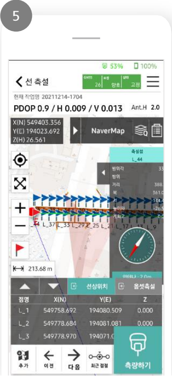
측설 선의 간격마다 측설 점 생성
