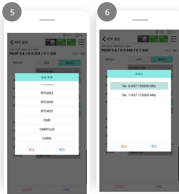
[방송 포맷 설정]
