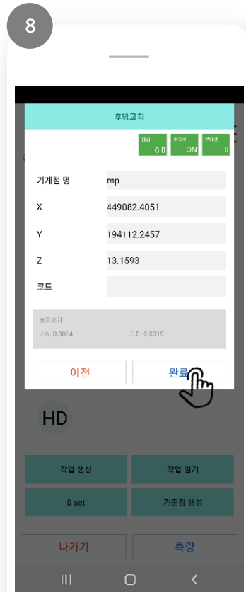
기계점 좌표가 계산되며 표준오차 N,E 값 확인 후 [완료] 클릭
