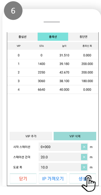
입력된 것을 확인 후 [생성] 클릭 - STA : 스테이션 정보 - 높이 : 계획고 - 종곡선 폭 : 종곡선의 길이 시점과 종점의 높이는 0값 입력
